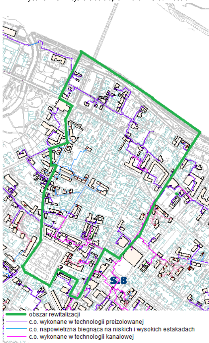
Rysunek 13. Miejska sieć ciepłownicza w Śródmieściu
